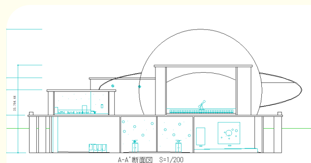
A-A' 断面図 S=1/200
